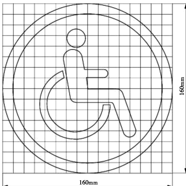
方格尺寸图
